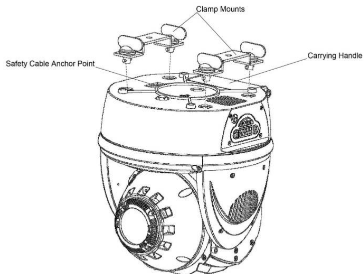
Figura 11. Soportes de abrazaderas, asa de transporte y anclaje de seguridad
