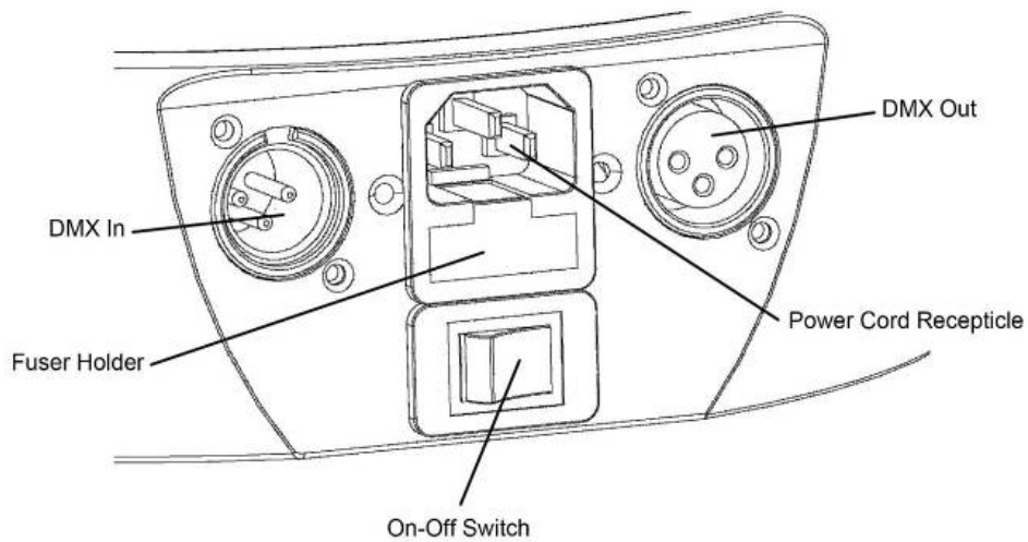
Figura 7. Primer plano del lado de los cables eléctricos/datos
