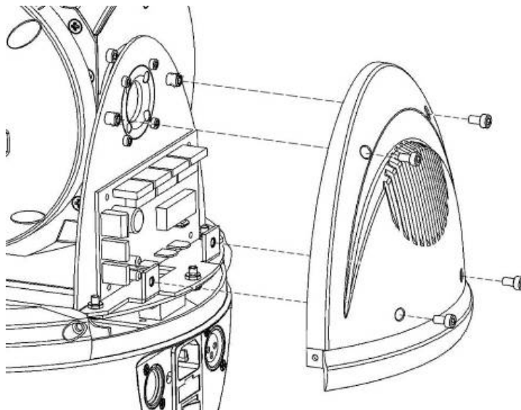
Figura 12. Extracción de las tapas del eje Y para su limpieza
