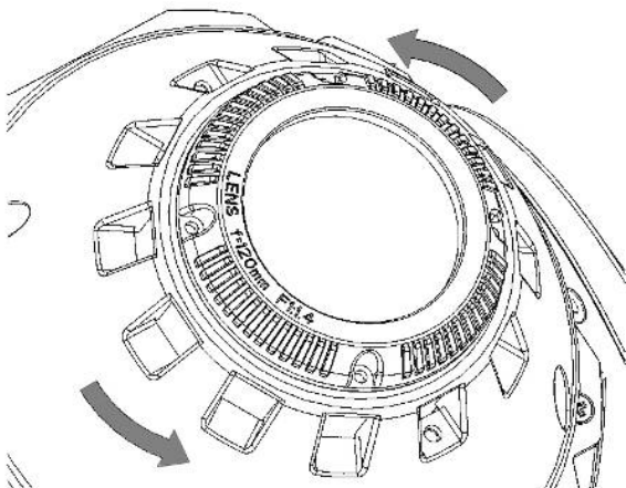
Figura 6. Apertura del objetivo y montaje del foco El anillo objetivo-foco puede girar en todas direcciones para poder enfocar el Merlin-Cpro lejos o cerca.
