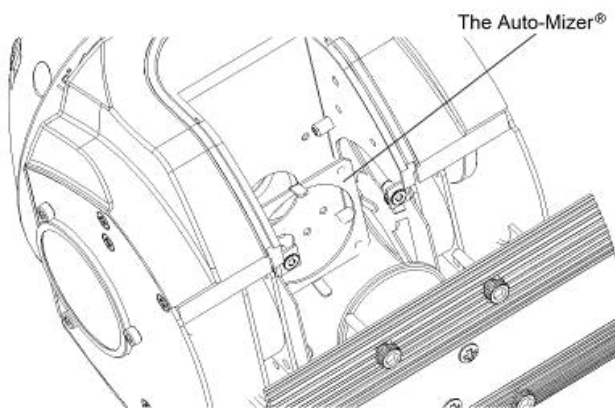
Figura 4.2. Vista transversal: Auto-Mizer® LAMP Esta sección transversal permite ver el Auto-Mizer LAMP dentro de la carcasa del Merlin-C. Está accionado por resorte, de modo que sujeta la lámpara en su base firmemente y de forma totalmente optimizada mientras el cabezal se mueve a su ritmo. ¡Ningún otro instrumento que utilice lámparas de tipo proyección ofrece esta extraordinaria característica!
