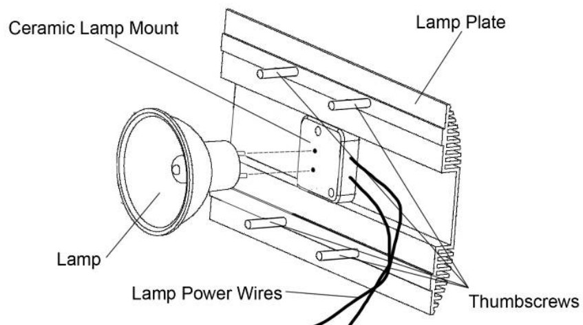
Figura 3. Colocación de la lámpara en el conector de cerámica
