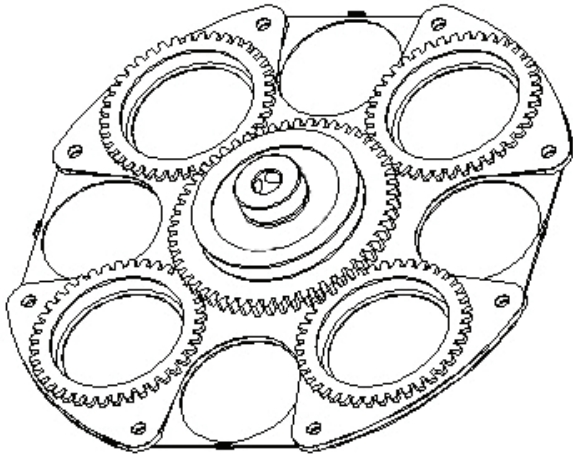
Figura 4.1. Vista transversal: Auto-Mizer® GOBOS Esta sección transversal permite ver el Auto-Mizer GOBOS dentro de la carcasa del Merlin-Cpro. Se trata de una fina rueda de gobos de 4 mm, indexable, sustituible, que hace que los engranajes de la rueda se muevan de forma óptima y fluida. Y está optimizado al máximo para el foco óptico, que ofrece una calidad de imagen muy buena.
