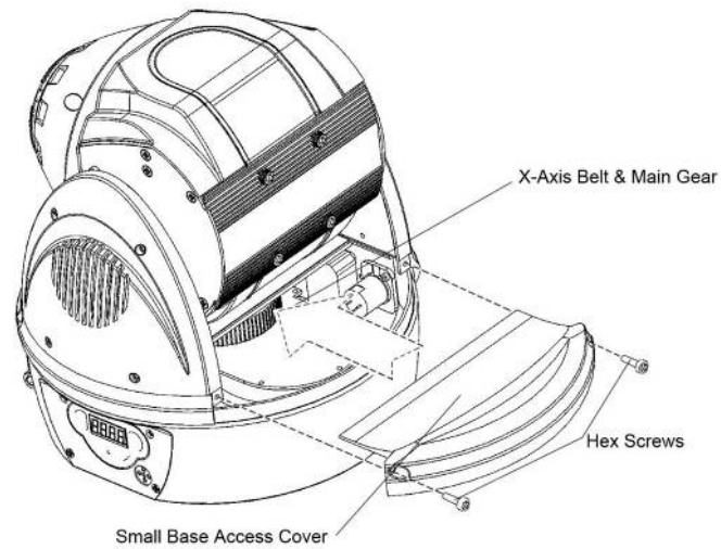
Figura 10. Extracción de las tapas de acceso a la base para limpiar y comprobar la correa del eje X.
