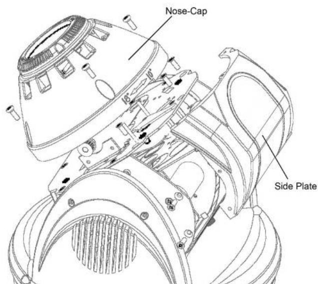
Figura 9. Extracción de las placas laterales y la tapa cónica para limpiar las rejillas, objetivos y comprobar la correa del eje Y, el regulador de luz/obturador y las ruedas de gobos y de colores
