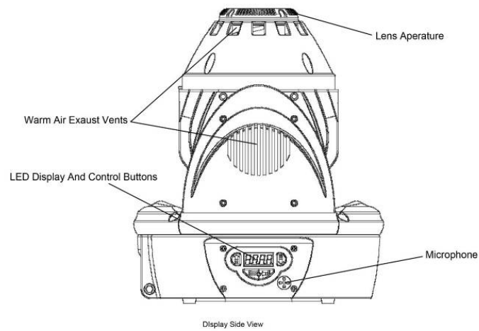
Figura 1. Vista del lado de la pantalla
