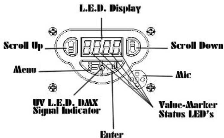
Figura 13. Sección de la pantalla LED LA PANTALLA LED
