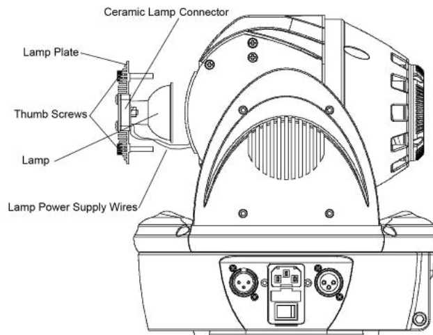
Figura 2. Extracción de la placa de la lámpara
